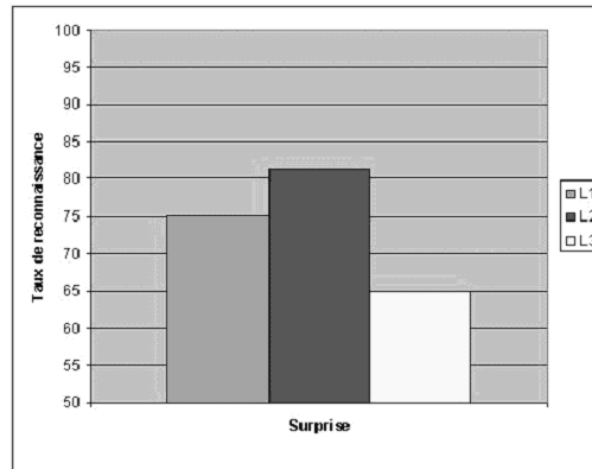
Figure 4.5: Impact des métriques utilisées (L1, L2 et L3) sur le taux de reconnaissance de l'émotion surprise.
